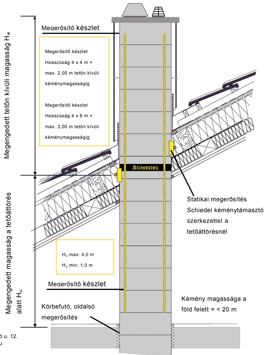
Szarufák közé történő elhelyezés
