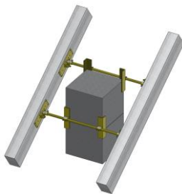
Szarufák közé történő elhelyezés
